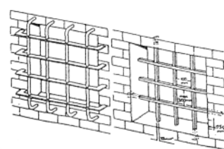
Példa a fixen beépíthető rács kialakítására
