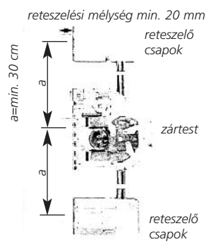
Több pontos zárás megoldása
